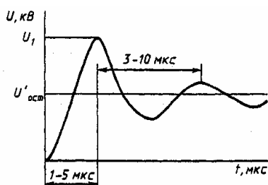
Рисунок Д.3. Форма грозовых импульсов, характерная для точек присоединения, проходящих через выводы силового трансформатора, рассматриваемая обмотка которого имеет связь с ВЛ (точки присоединения з, з', и на рисунке Д.1)
