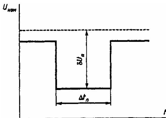
Рисунок Б.2. Провал напряжения
