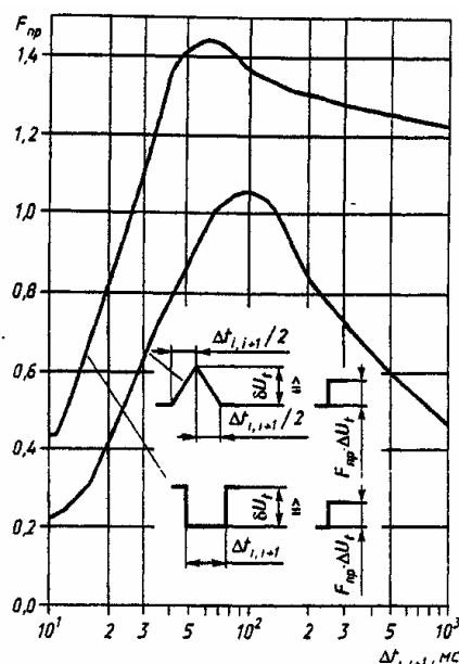
Рисунок В.2. Коэффициент приведения F_{\text{пр}} для прямоугольных и треугольных периодических колебаний напряжения
