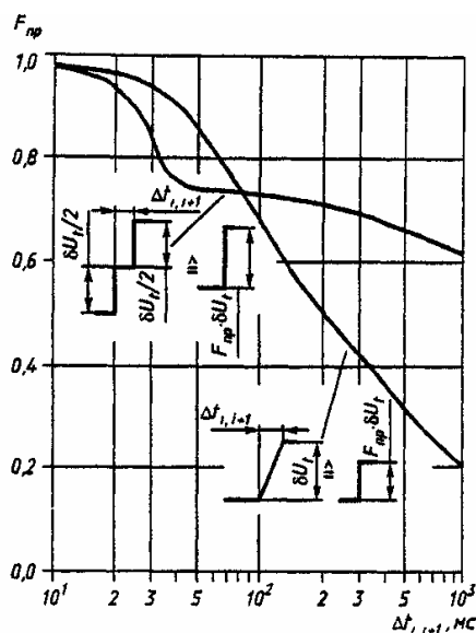
Рисунок В.1. Коэффициент приведения F_{\text{пр}} для периодических колебаний напряжения, имеющих двухступенчатую и пилообразную
